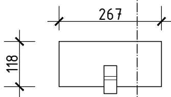
Presek kroz gorionik 1-1
